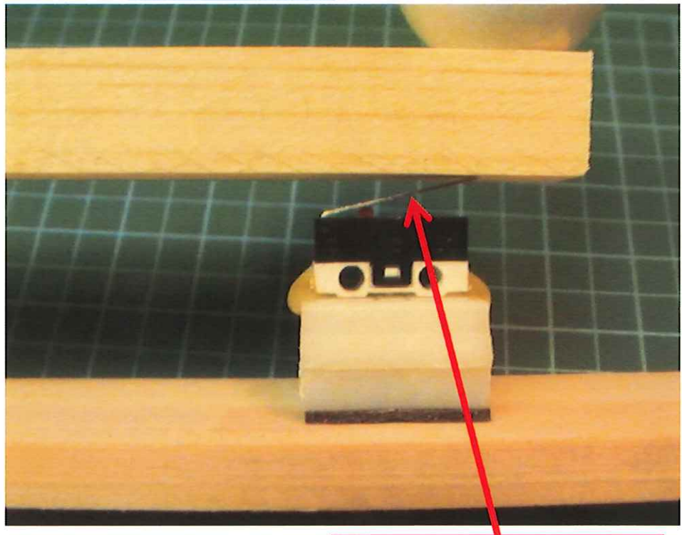
⑥スイッチ
